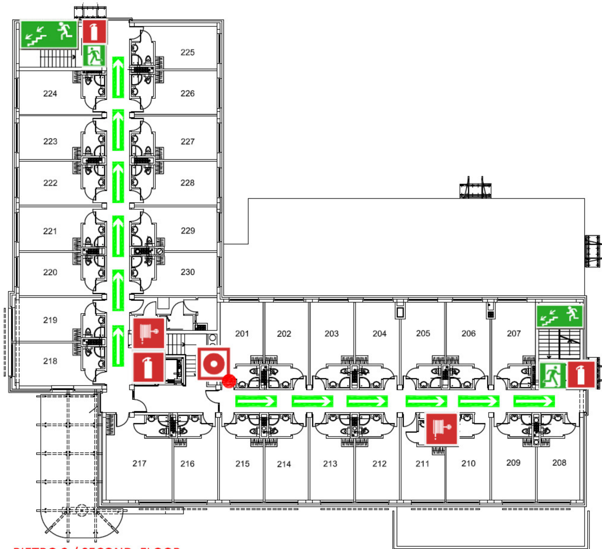
PIĘTRO 2 / SECOND FLOOR
